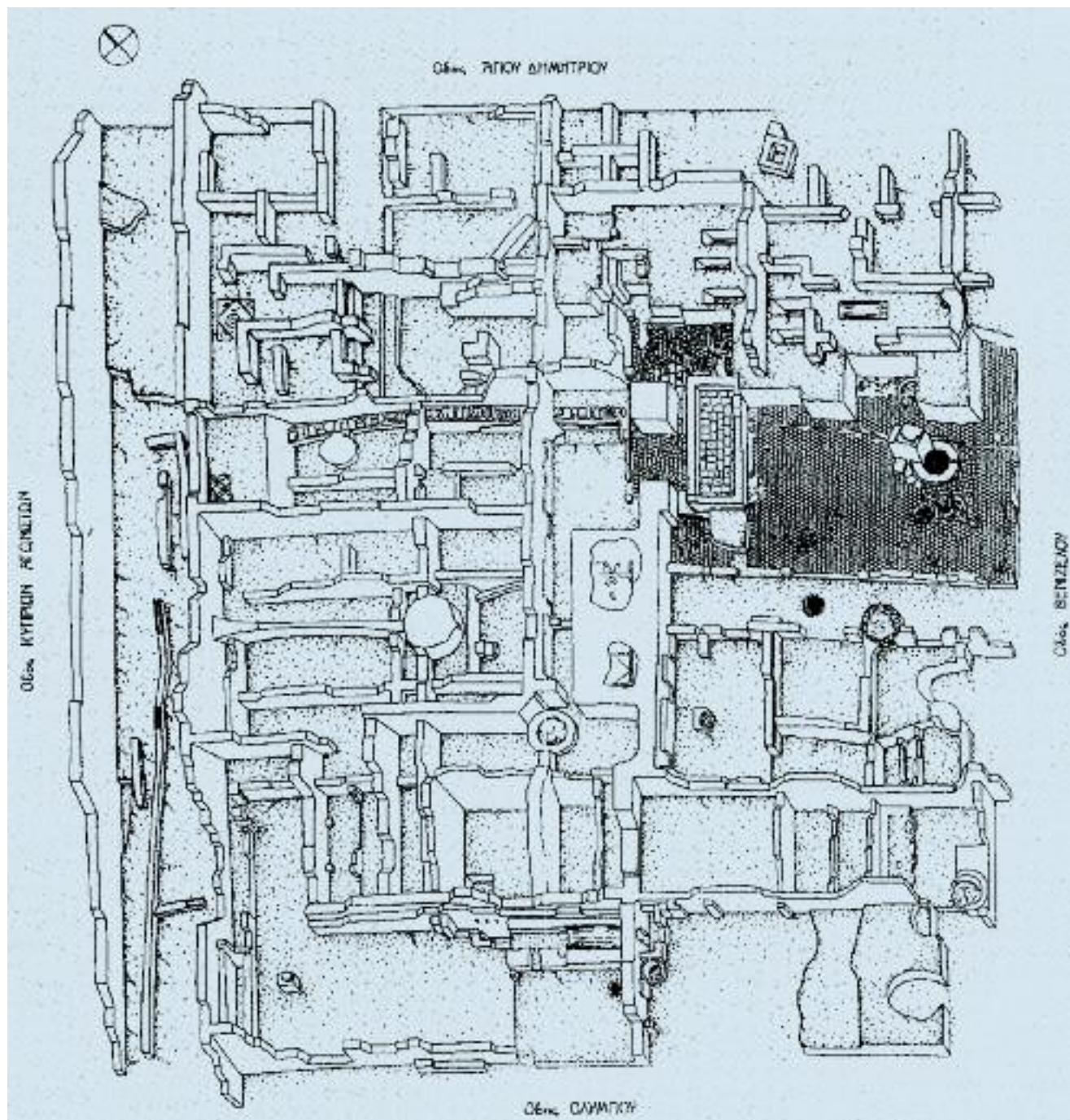
Εικ. 2. Αξονομετρικό των κτισμάτων της ανασκαφής στην Πλατεία Διοικητηρίου (φυλλάδιο, Θεσσαλονίκη Πολιτιστική Πρωτεύουσα της Ευρώπης 1997).
